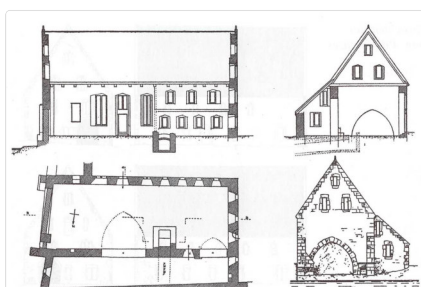
Die Walkmühle. Grundriß, Ansicht und Schnitte
