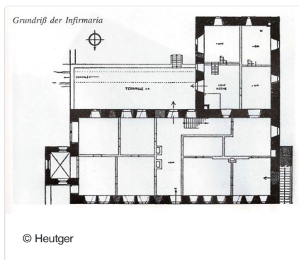
Grundriß des ehemaligen Siechenhauses (unten = Norden) aus HEUTGER (1999: 89)
